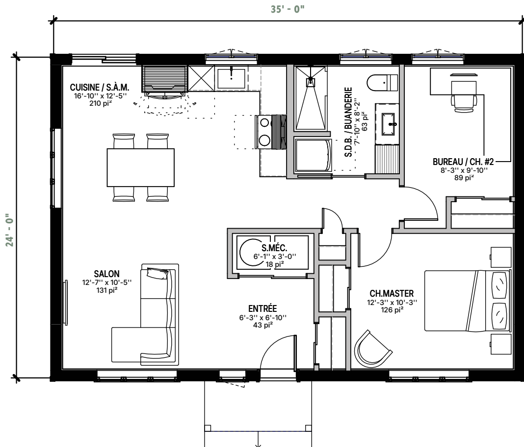
REZ-DE-CHAUSSÉE
