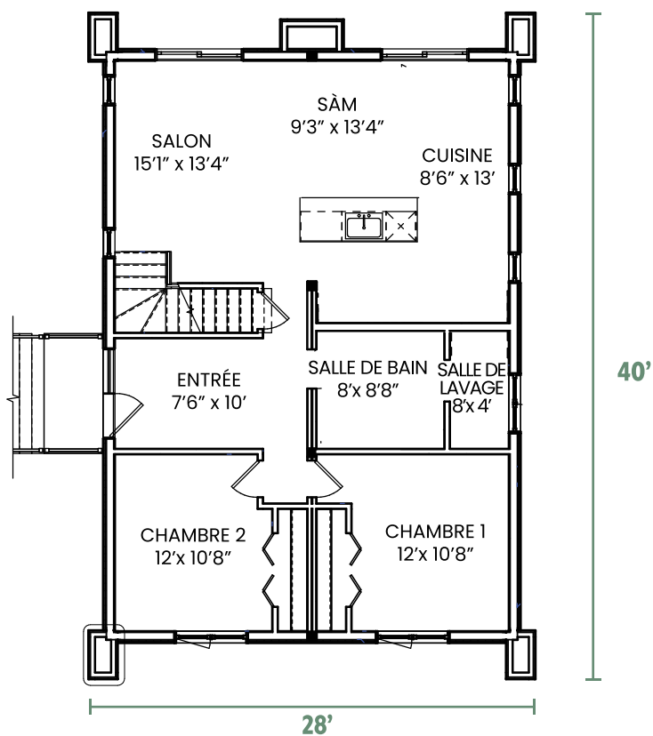
REZ-DE-CHAUSSÉE
