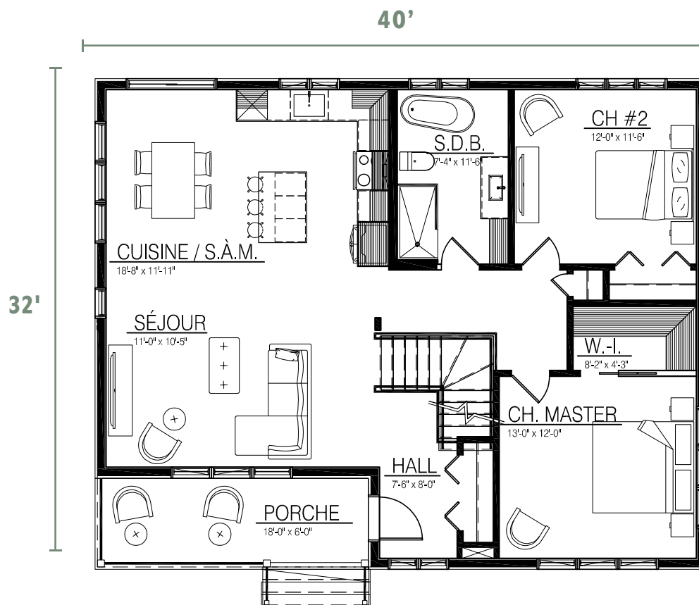
REZ-DE-CHAUSSÉE
