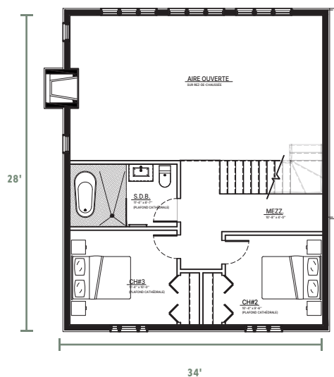
2E ETAGE
